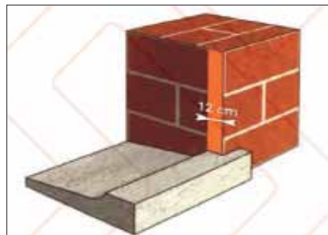
شکل ۴۰ آماده‌سازی سطوح یک درگاه ساخته شده از بلوک یا آجر سوراخ‌دار با تکیه‌گاه پیش ساخته در حالت نصب توکار
